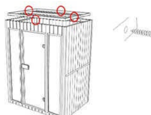
Upevnenie stropu
